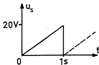
Figur 4.7 a, b. Elektronisk voltmeter och voltmeters svepspänning.
