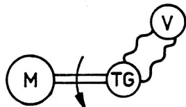
Figur 4.2 a. Analog varvtalsmätning med takometergenerator. Spänningen är analog med varvtalet.
