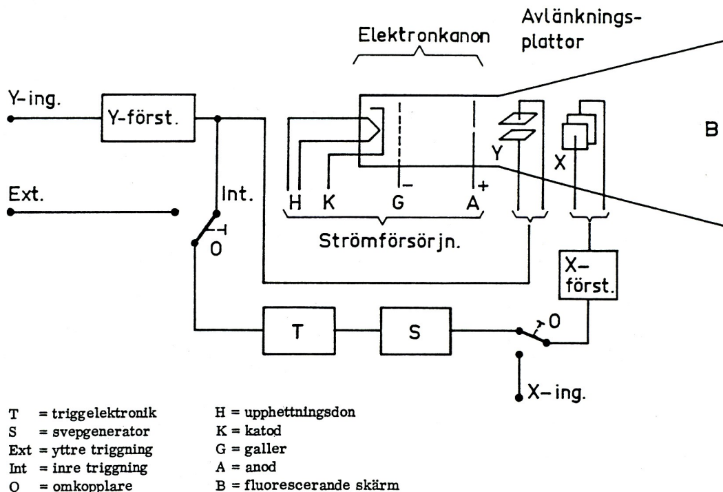
Figur 4.11. Oscilloskopets uppbyggnad
