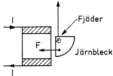
Figur 4.5. Vridjärnsinstrument. Utslaget proportionellt mot strömmens effektivvärde.
