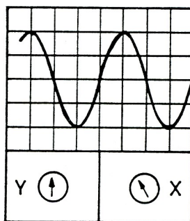
Figur 4.12 c. Oscilloskopbild 2 Inställning:
