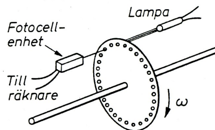
Figur 4.2 b. Digital varvtalsmätning med hålskiva, fotocell och räknare. Antalet pulser under en viss tid räknas.
