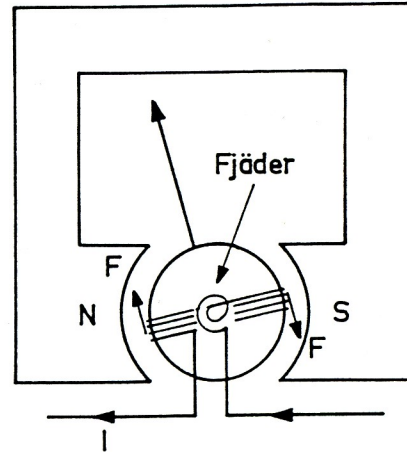
Figur 4.4. Vridspoleinstrument. Utslaget proportionellt mot strömmens medelvärde.
