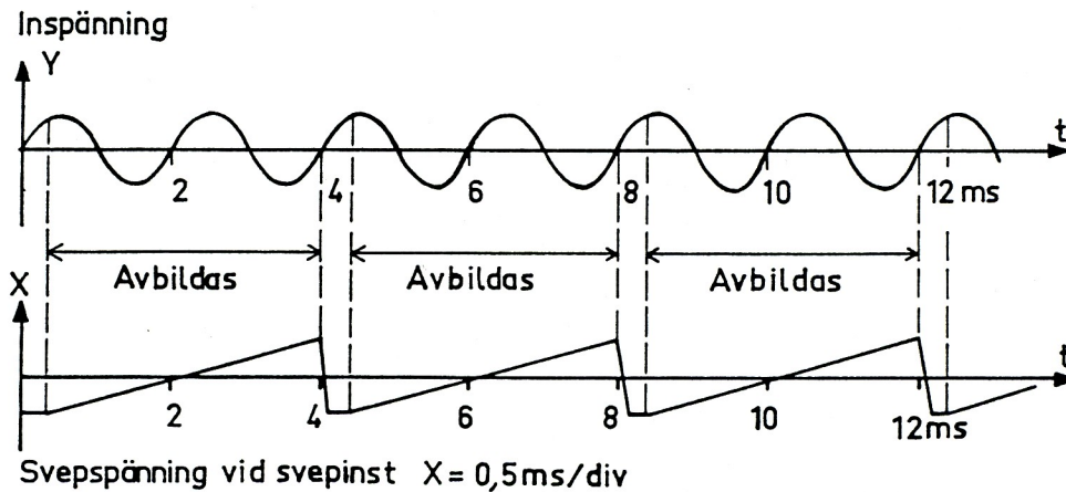
Figur 4.13. Principen för trigging
